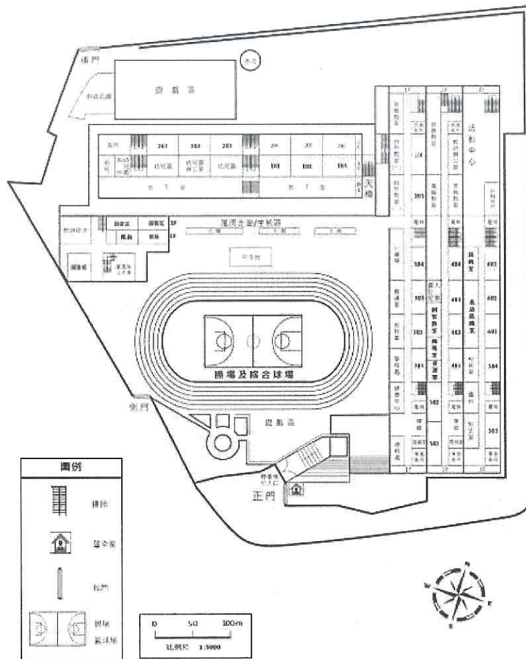
桃園市龜山區樂善國民小學 111 學年度校舍平面圖
